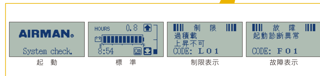
下部操作盤
